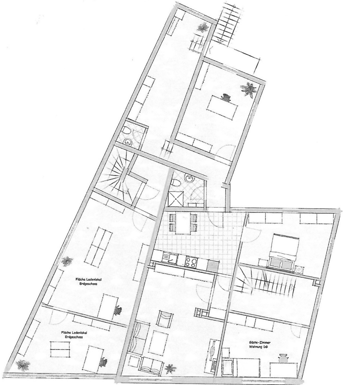
Wohnung 1 / 1. OG
